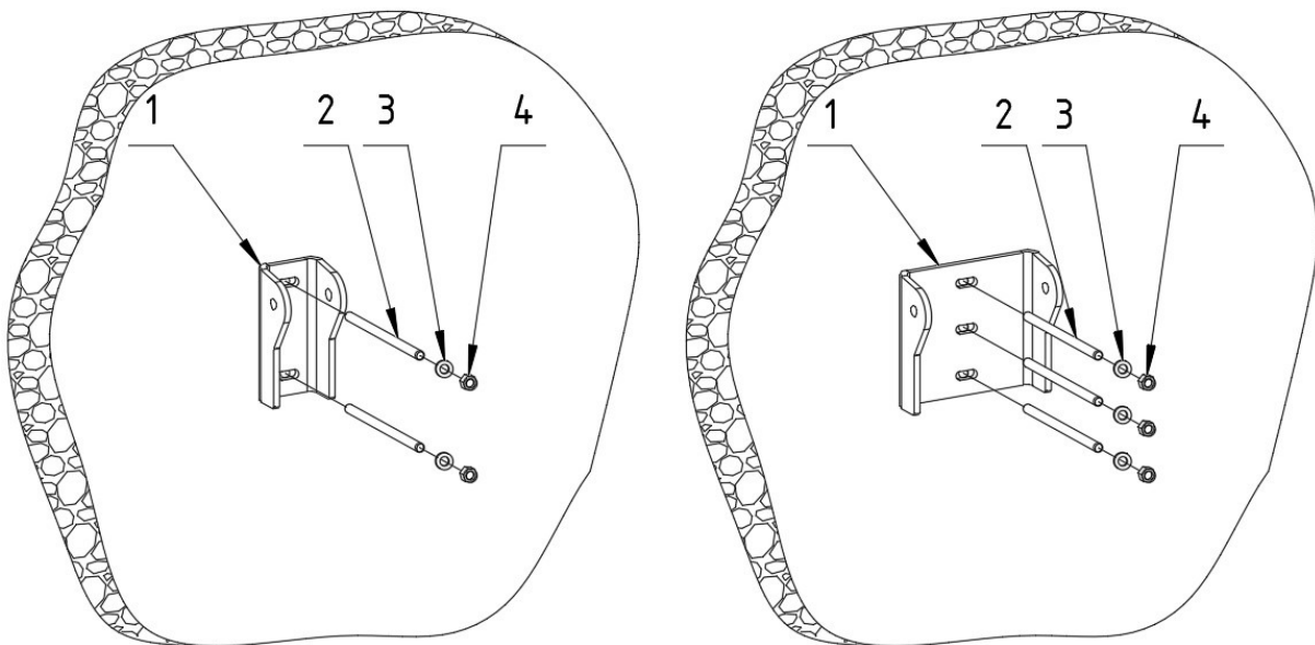
Zeichn. 40. Montageart des hinteren Führungsschienehalters (links – Einzel-Führungsschienehalter, rechts – Doppel-Führungsschienehalter): 1 – hinterer Führungsschienehalter (Einzel / Doppel), 2 - Verankerung (Fixierendes Element), 3 - Unterlegscheibe, 4 - Mutter.
