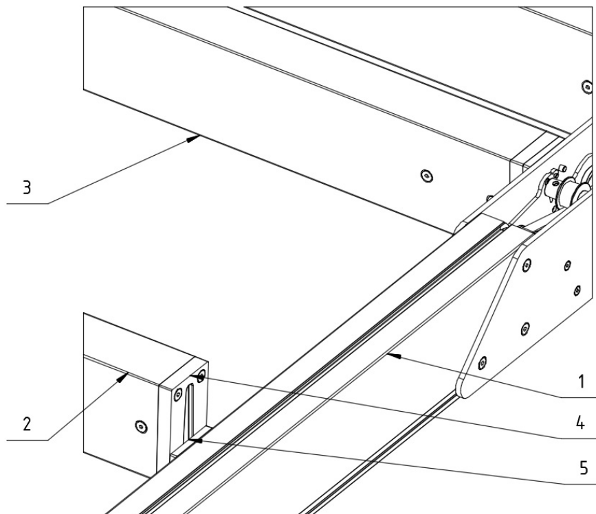
Zeichn. 13b. Montage der Verstärkungen: 1 - Führungsschiene, 2 - Verstärkung (Vorne), 3 – Verstärkung (hinten) , 4 – Scherpen-Gegenstück, 5 - Scherpe.
