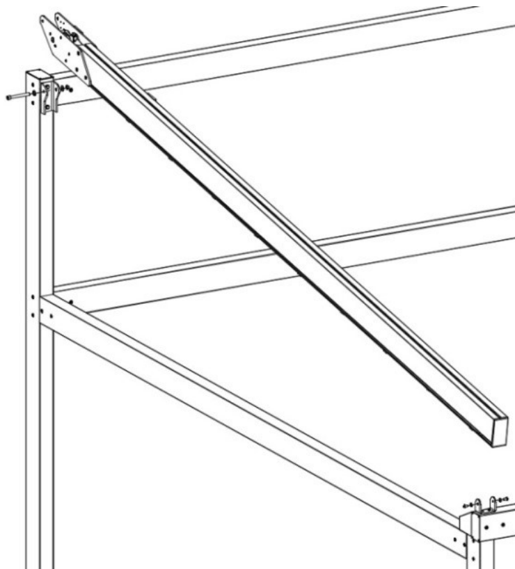
Zeichn. 10. Montage der Führungsschiene.
